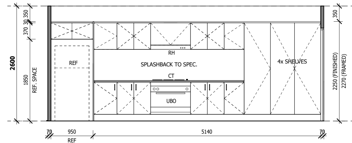
ELEVATION K1
