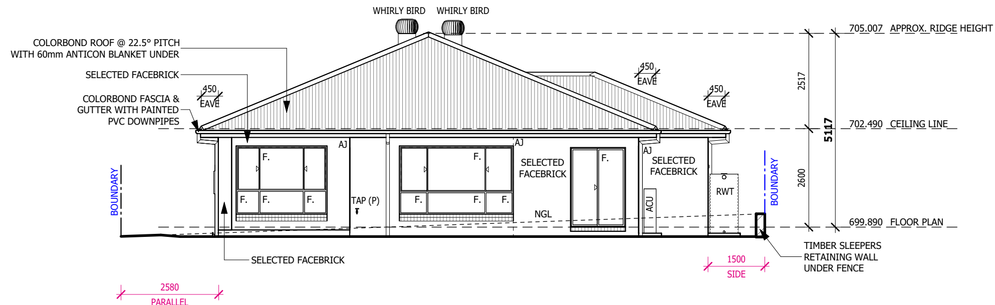
ELEVATION 3
