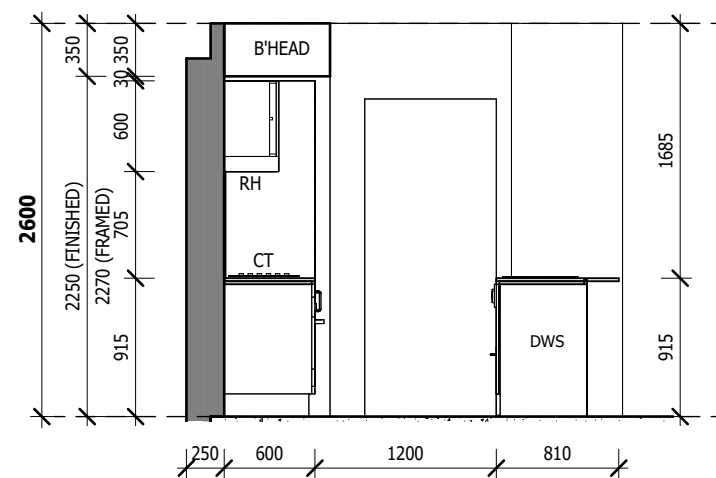
ELEVATION K2
