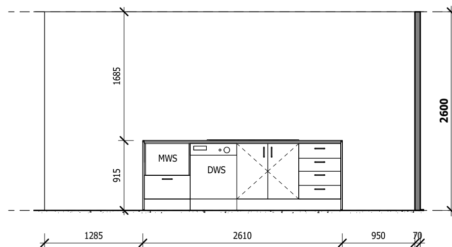
ELEVATION K3
